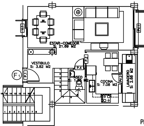
PLANTA PRIMERA
