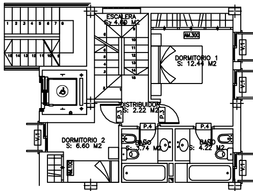
PLANTA PRIMERA
