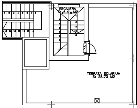
PLANTA TORREON
